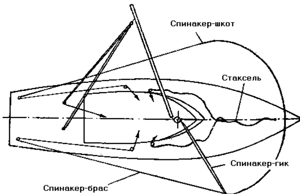
Рис. 48. Такелаж спинакер-гика
