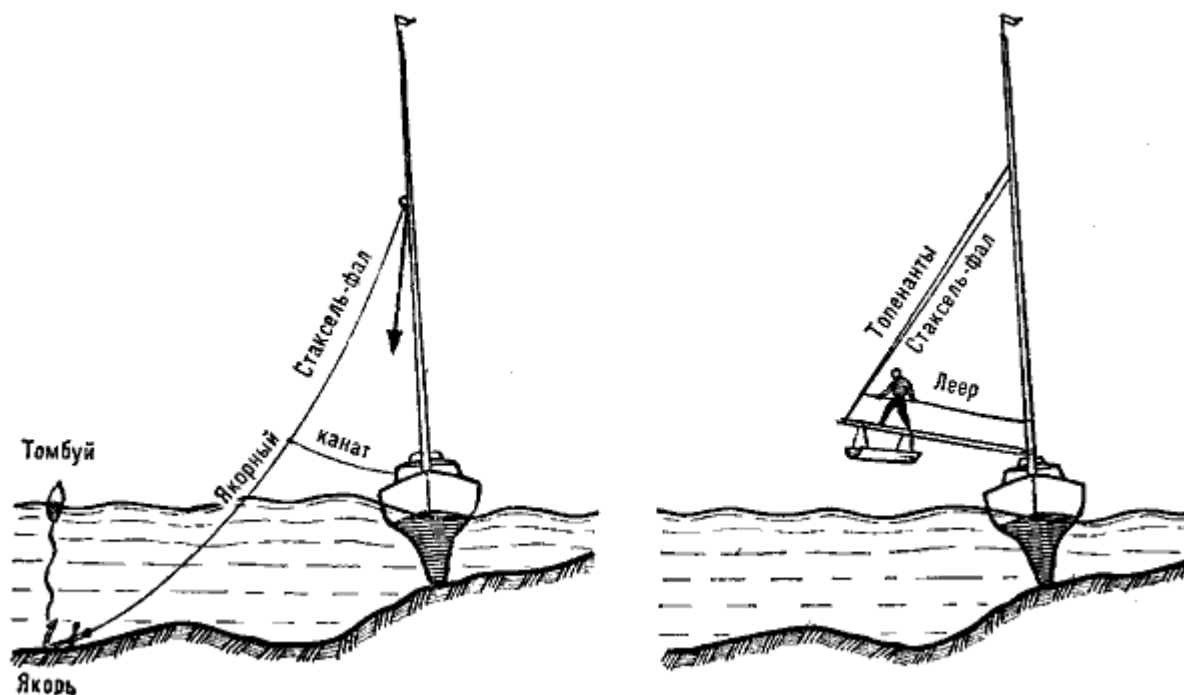
Рис. 139 Способы закрепления яхты на мели
