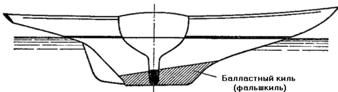
Рис. 4. Килевая яхта
