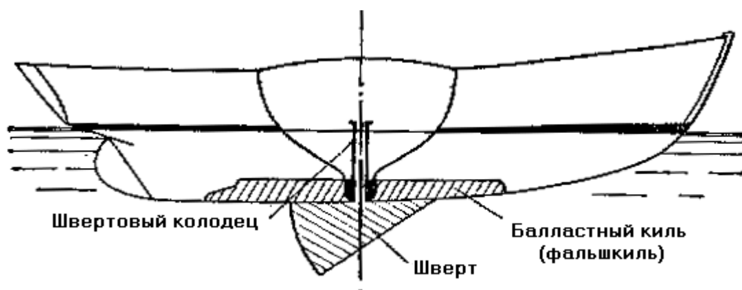
рис. 6. Яхта-компромисс
