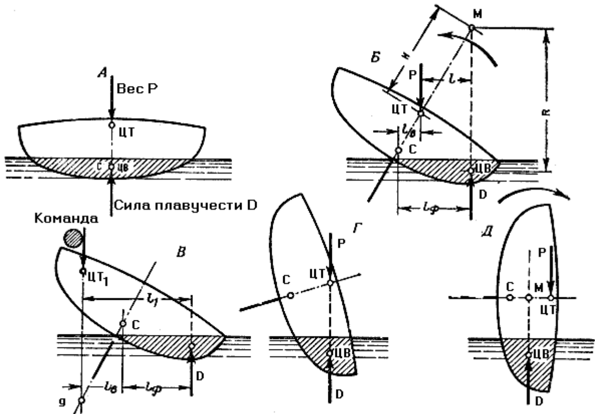
Рис. 78. Остойчивость швертбота
