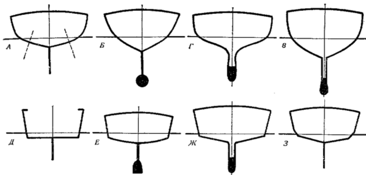
Рис. 9. Формы мидель-шпангоутов.
