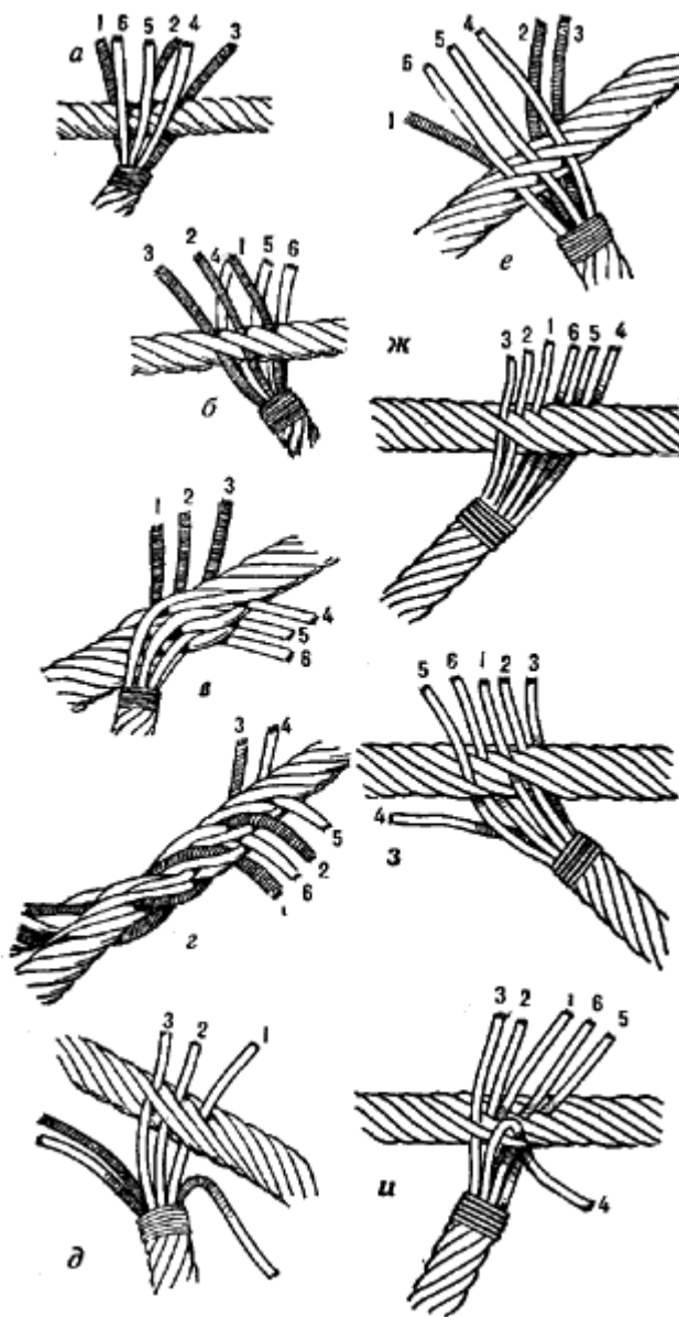
Рис. 66. Огон на растительном тросе
