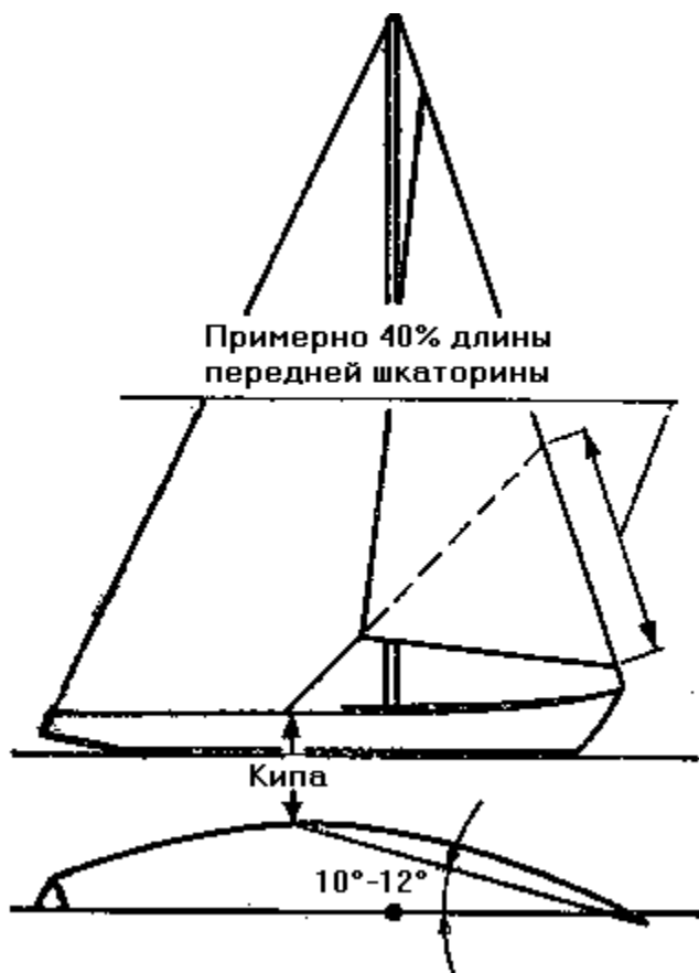
Рис. 46. Проводка стаксель-шкотов
