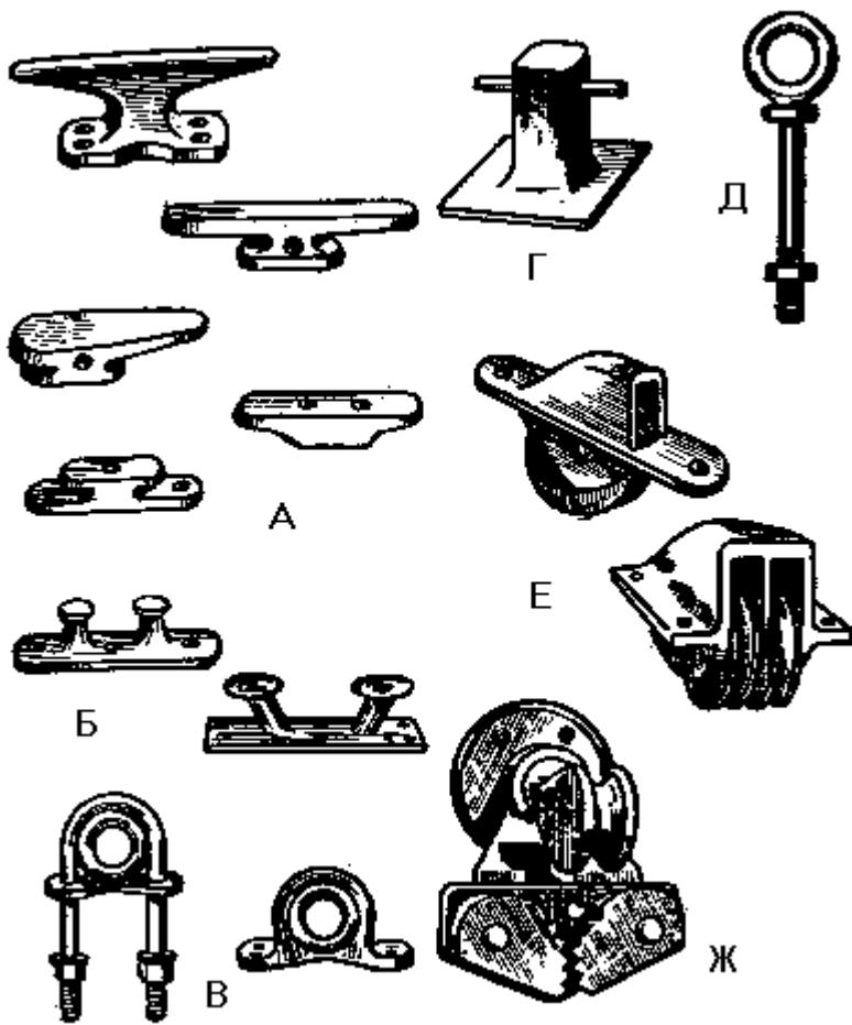
Рис. 50. Дельные вещи:
