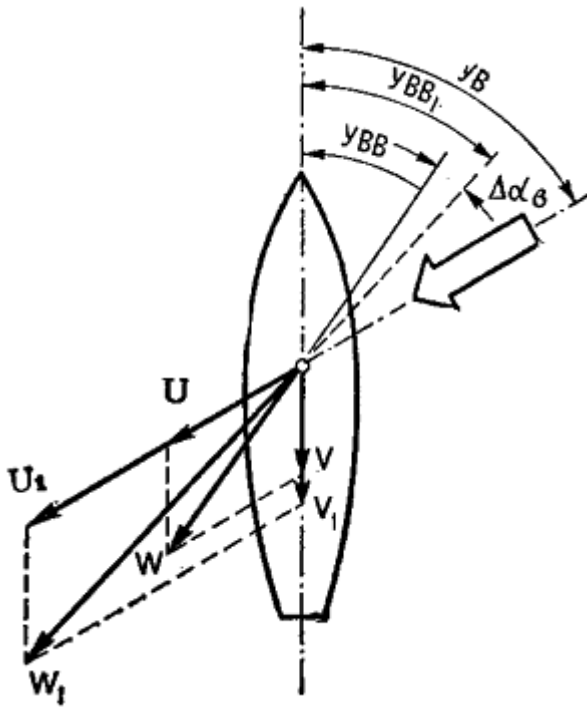
Рис. 91. При слабом ветре выпел отклоняется больше, чем при сильном
