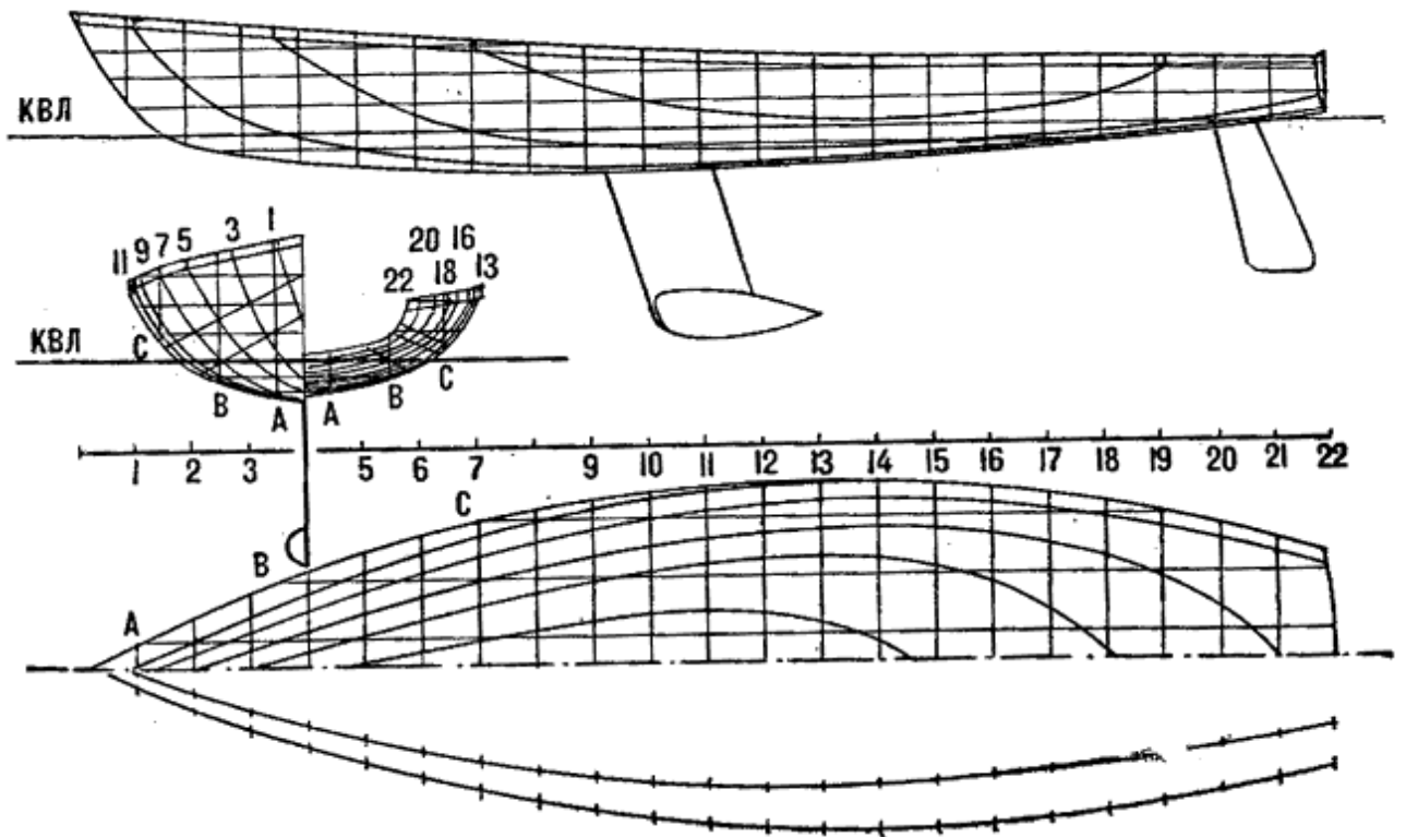
Рис. 85. Теоретический чертеж килевой яхты класса «Темпест»
